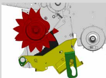
Drop Floor in posizione di lavoro.
