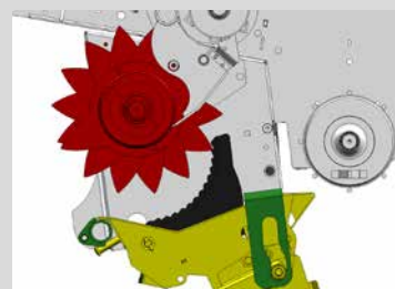
Drop Floor in posizione completamente abbassata.
